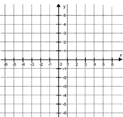
Wykres funkcji h \circ f \circ g .
